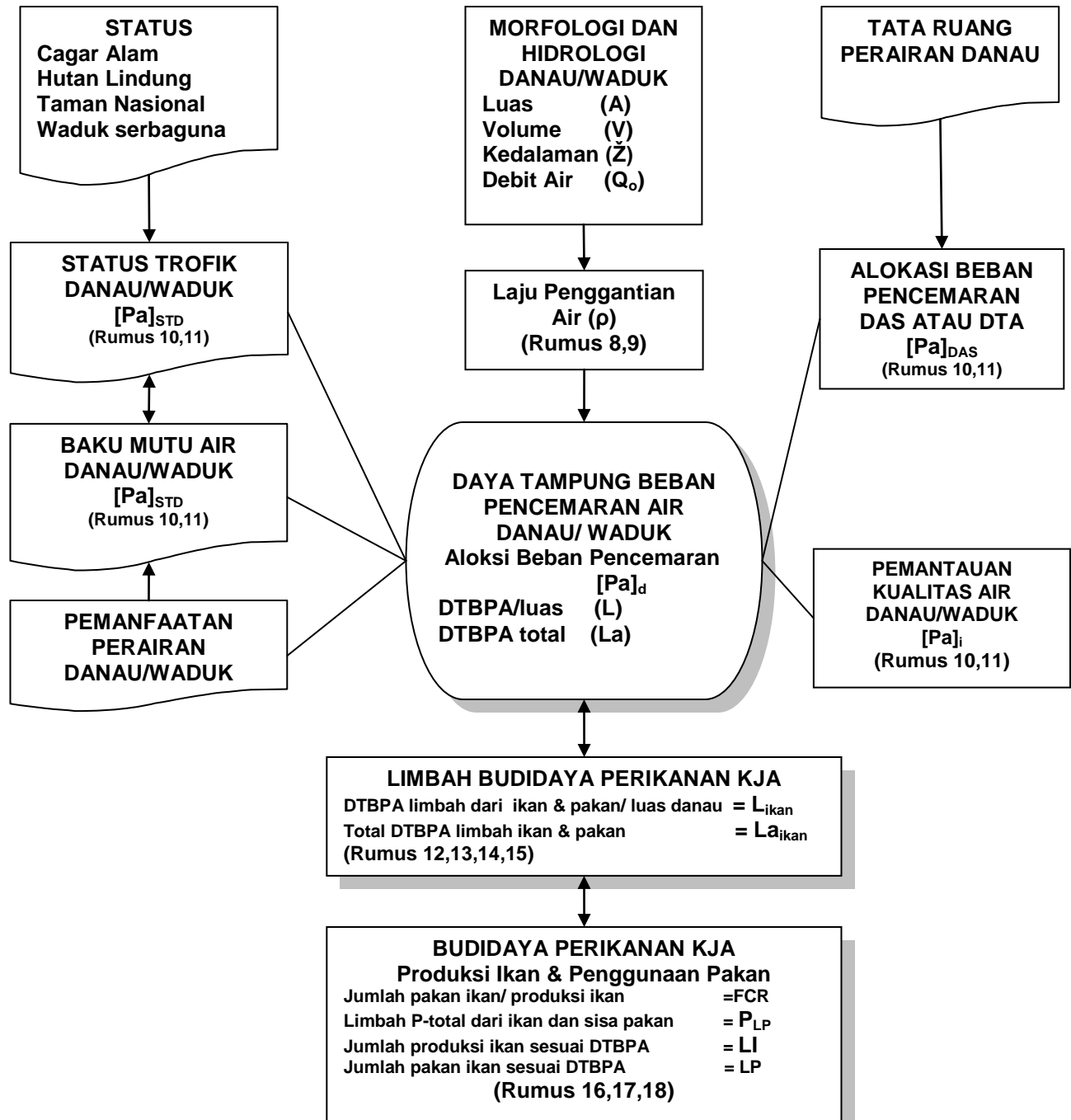
Gambar 2. Model dan Perhitungan Daya Tampung Beban Pencemaran Air Danau dan/atau waduk Untuk Limbah Budidaya Perikanan 8
