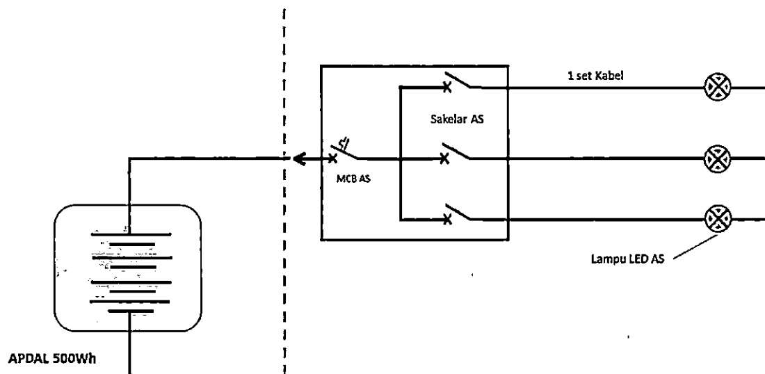
Gambar 4a. Diagram Garis Konfigurasi IRAS
