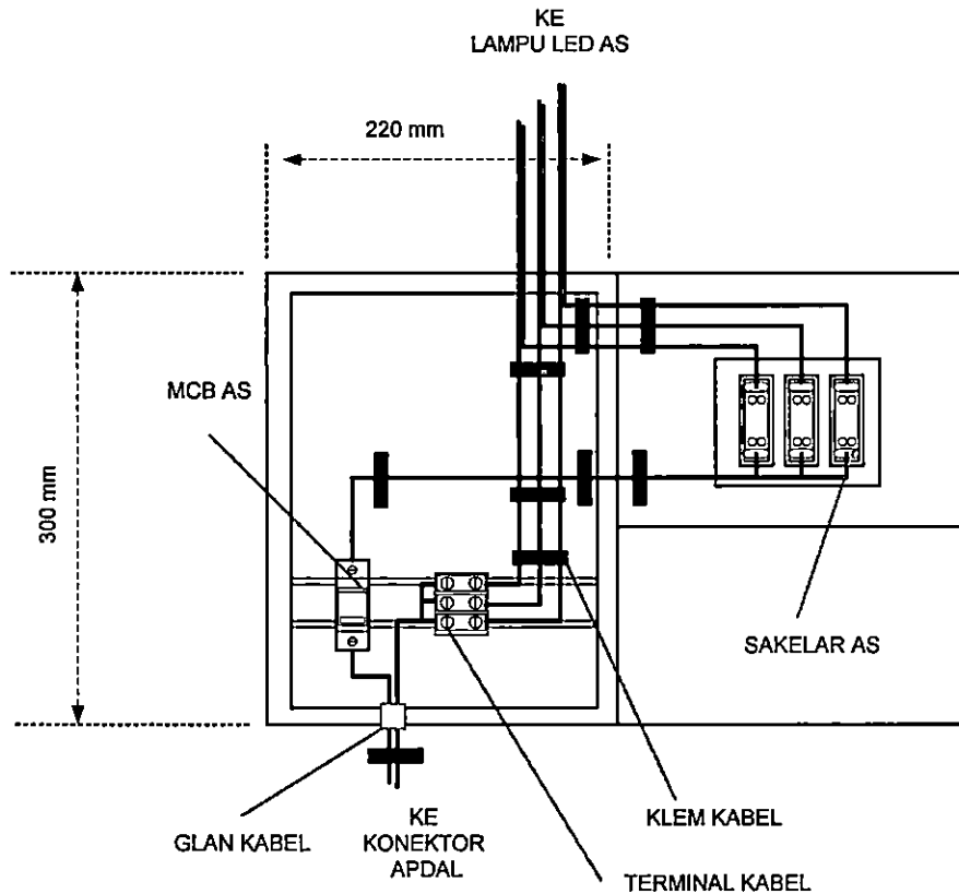
Gambar 4b. Diagram Tata Letak ( Lay Out ) Konfigurasi Perengkapan Hubung Bagi dan Kendali (PHBK) dan IRAS
