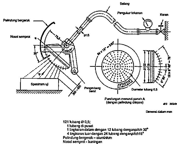
Gambar 3. Gawai Genggam untuk Memverifikasi Proteksi terhadap Semprotan dan Percikan Air (Nozsel Semprot)
